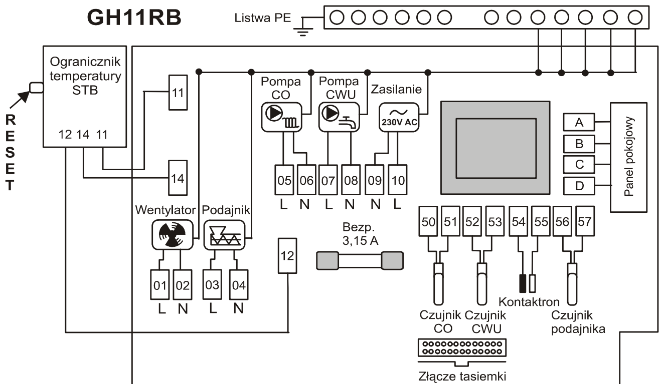
Rys. 2 Schemat podłączenia urządzeń i czujników do regulatora GH11RB
