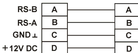
Rys. 1 Schemat podłączenia panelu pokojowego GA01HA do sterownika GH11RB
