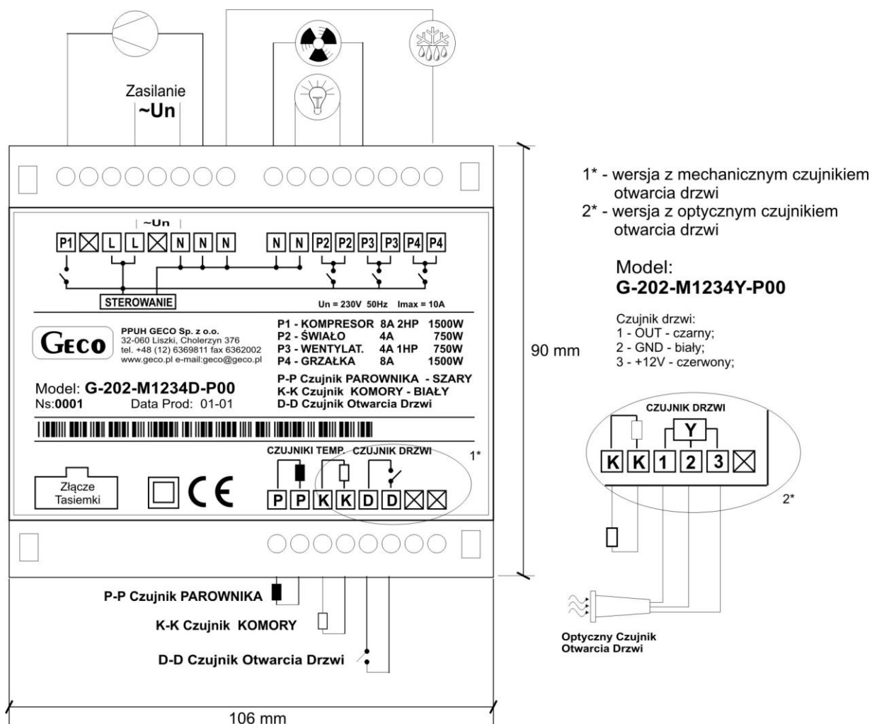
Rys. 2 Schemat podłączenia urządzeń do głównego modułu sterownika.
