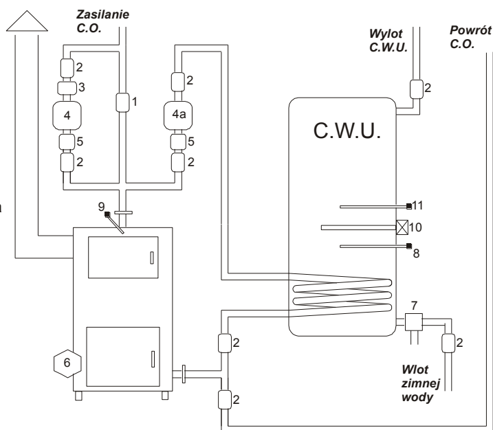
Rys. 2 Schemat blokowy instalacji C.O. w układzie z pompą obiegową oraz pompą ładującą bojler C.W.U.
