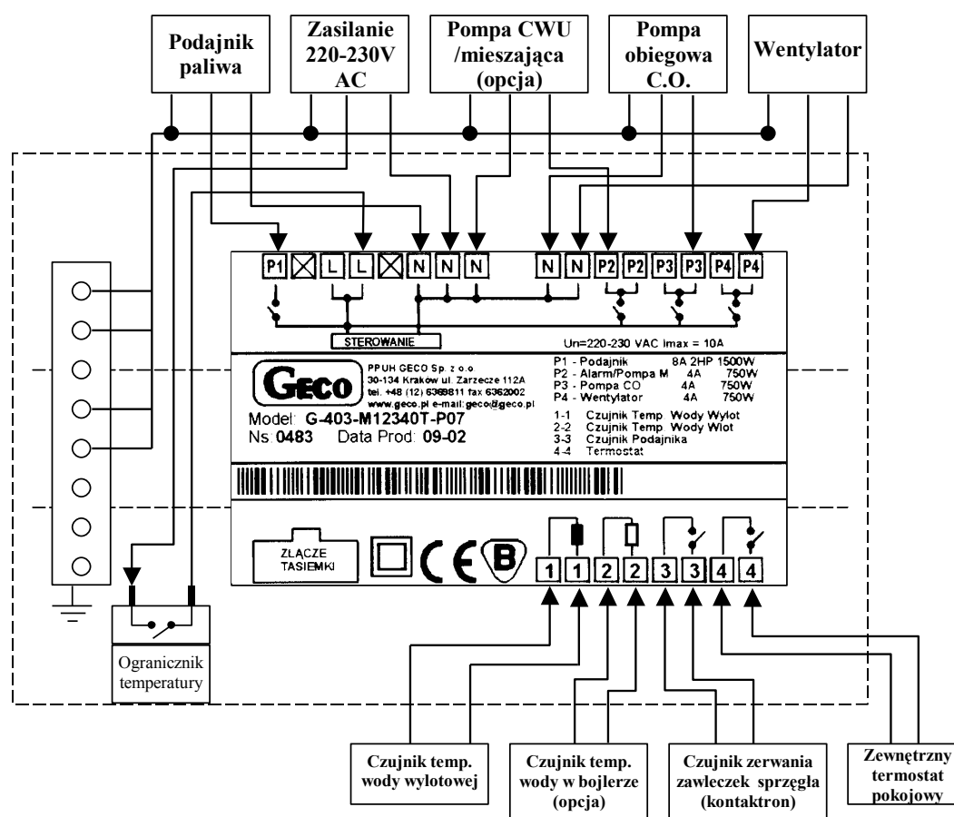
Rys. 3 Schemat podłączenia urządzeń i czujników do regulatora G-403-P07.
