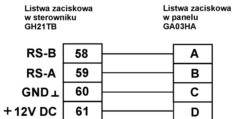
Schemat podłączenia panelu pokojowego GA03HA do sterownika GH21TB
