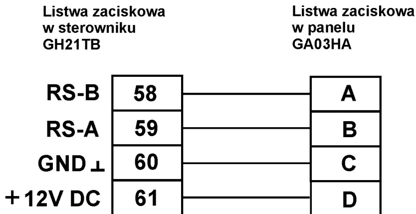
Rys. 12.1 Schemat podłączenia panelu pokojowego GA03HA do sterownika GH21TB
