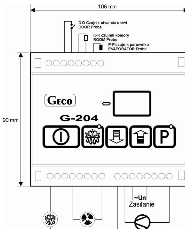
Rys. 3 Schemat podłączenia urządzeń do głównego modułu sterownika (opcja bez światła).
