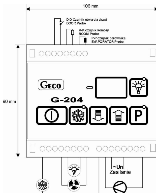
Rys. 2 Schemat podłączenia urządzeń do głównego modułu sterownika (opcja ze światłem).
