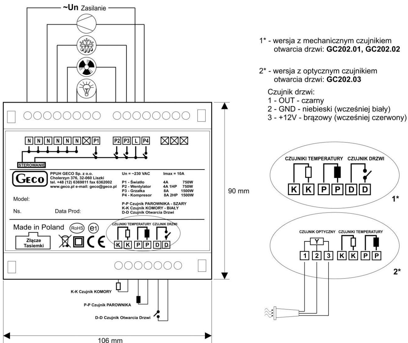
Rys. 2 Schemat podłączenia urządzeń do głównego modułu sterownika.
