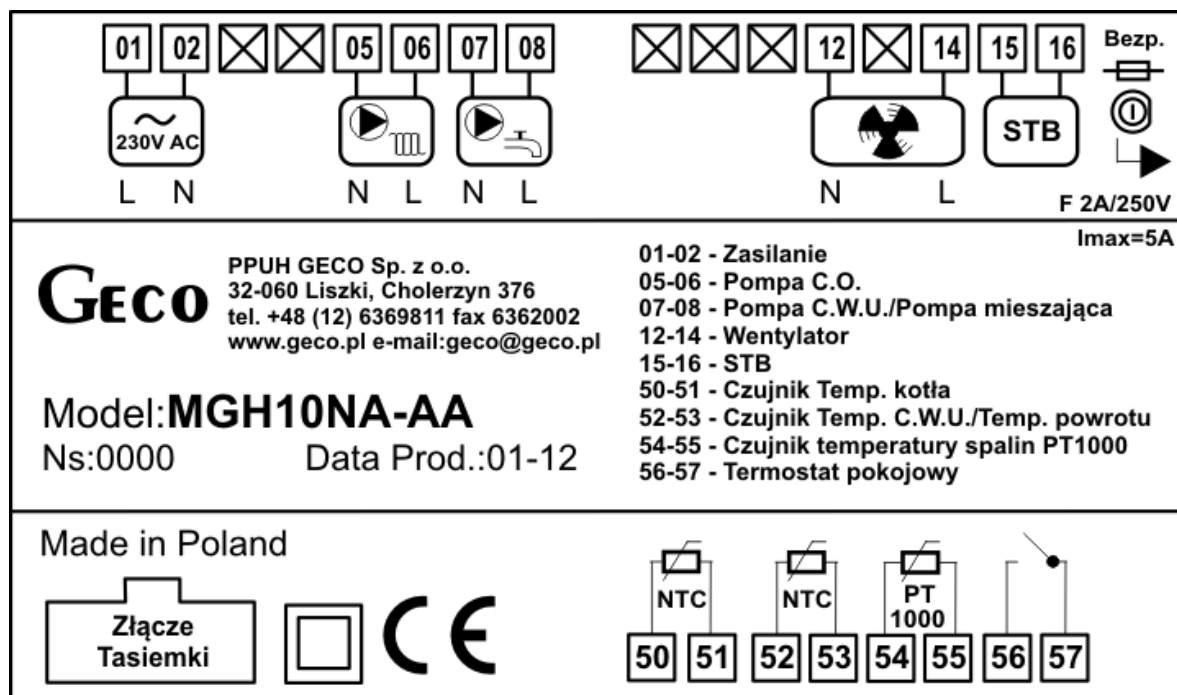
Rys. 1 Schemat podłączenia urządzeń i czujników do regulatora GH10NA.
