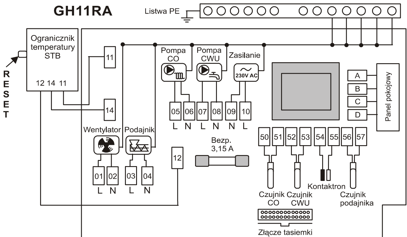
Rys. 2 Schemat podłączenia urządzeń i czujników do regulatora GH11RA
