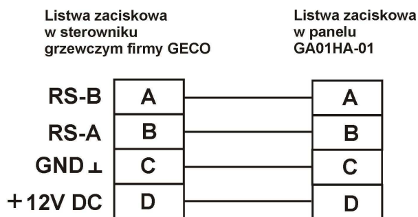
Rys. 1 Schemat podłączenia panelu pokojowego GA01HA do sterownika GH11RA
