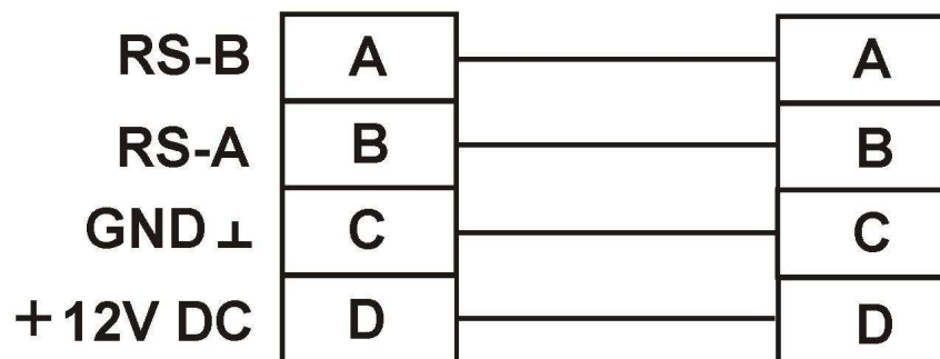
Rys. 1 Schemat podłączenia panelu pokojowego GA01HA do sterownika GH11NA
