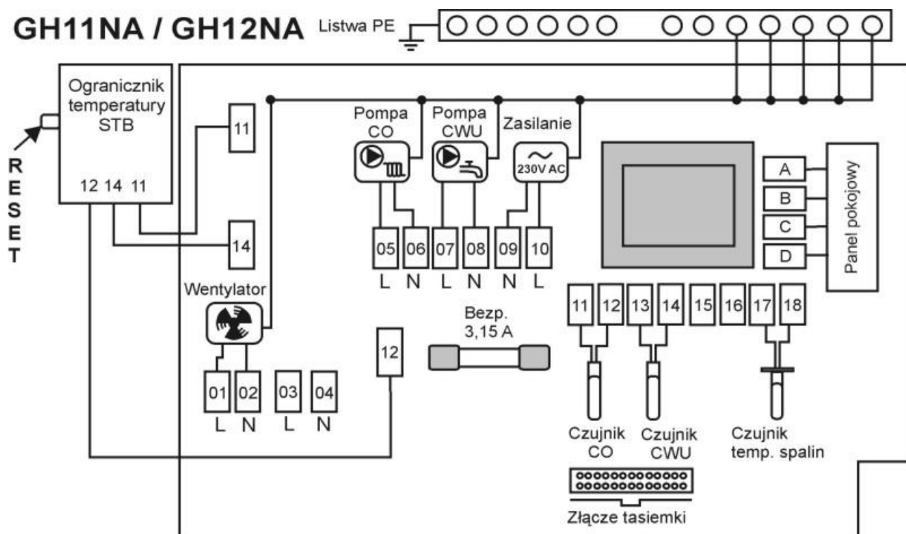
Rys. 2 Schemat podłączenia urządzeń i czujników do regulatora GH11NA.
