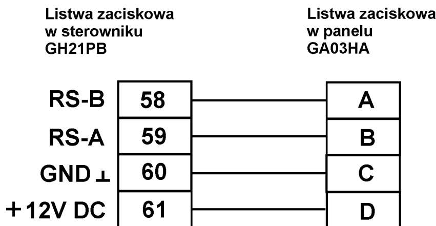
Schemat podłączenia panelu pokojowego GA03HA do sterownika GH21PB
