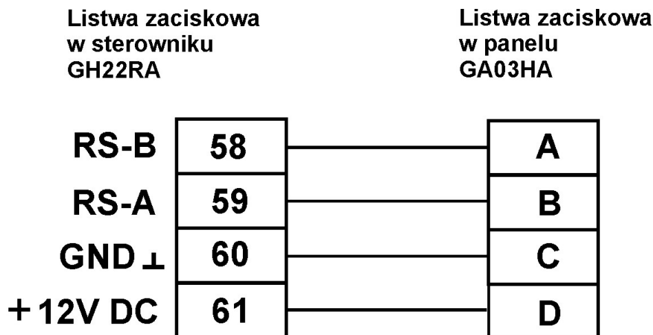
Schemat podłączenia panelu pokojowego GA03HA do sterownika GH22RA
