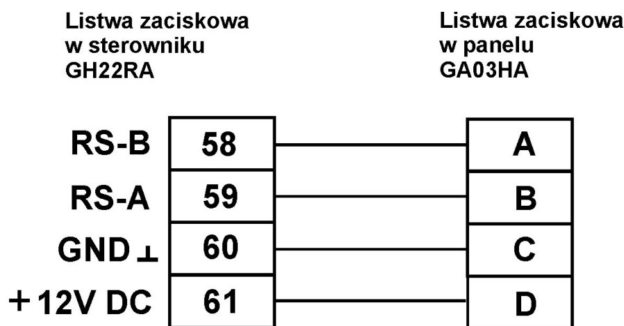
Rys. 12.1 Schemat podłączenia panelu pokojowego GA03HA do sterownika GH22RA
