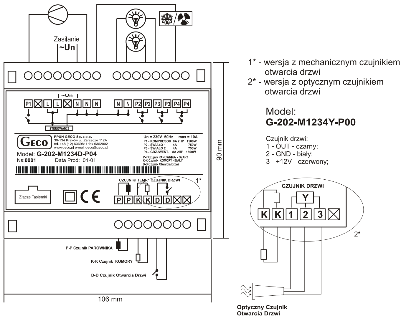
Rys. 2 Schemat podłączenia urządzeń do głównego modułu sterownika.
