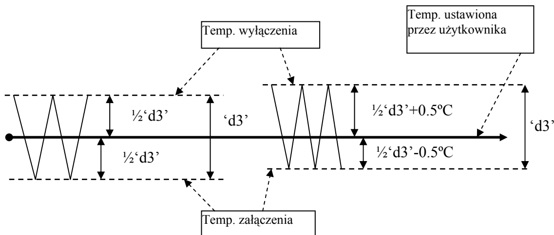
Rys. 1. Zasada działania histerezy.
